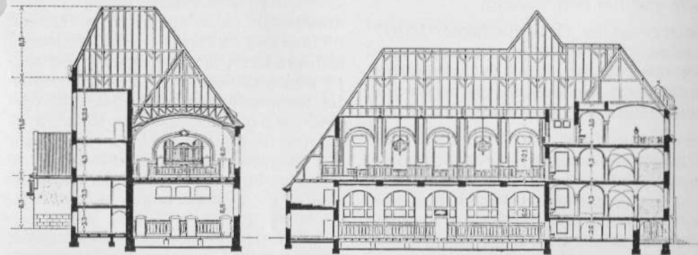
Abb. 1. Schnitt A B.
